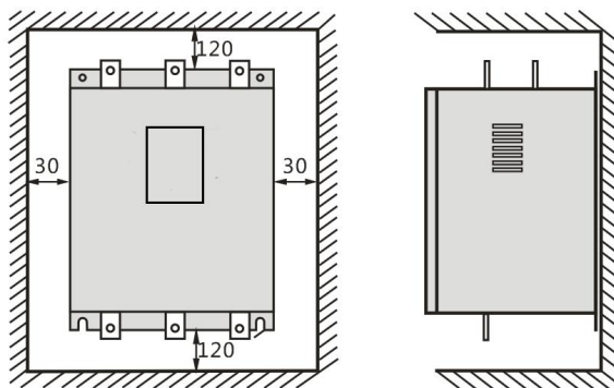
图 4.1 预留安装空间（示意图）
