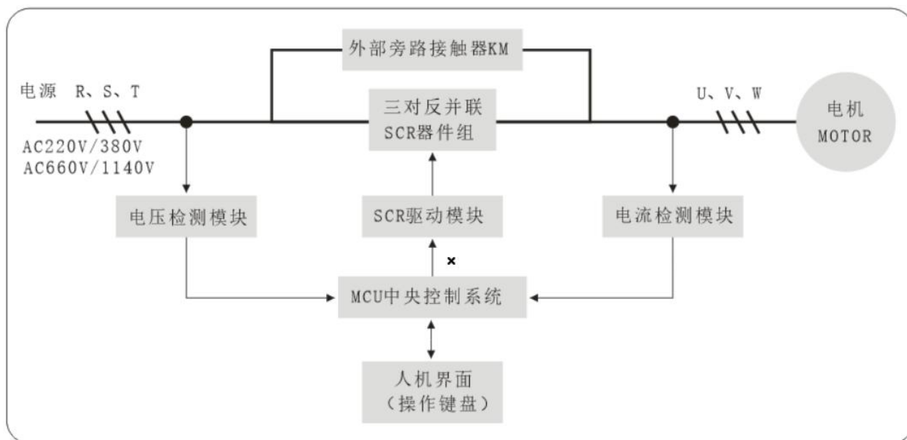
图 5.1 工作原理框图
