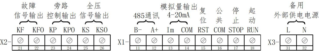
图 5.3 外控端子图
