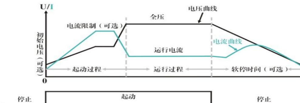
软起/软停的电压和电流特性曲线
